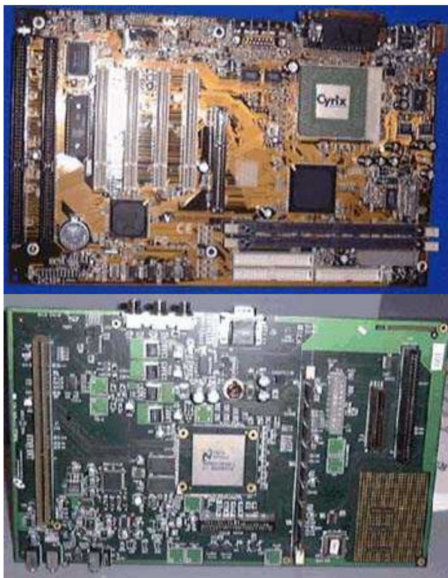
Placas Mãe usando o Cyrix Media Gx
