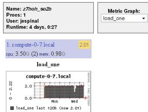
Figura 11. Información individual de un proceso en ejecución con SGE
