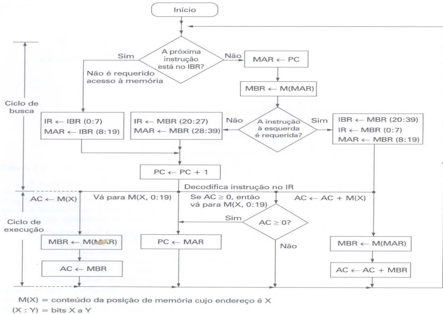
Figura 2.4 Fluxograma parcial da operação do IAS.
