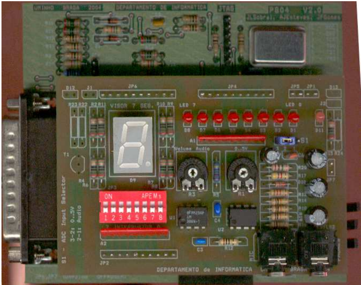
Figura 24: Painei do PG04 versão 2 ligado à placa principal.
