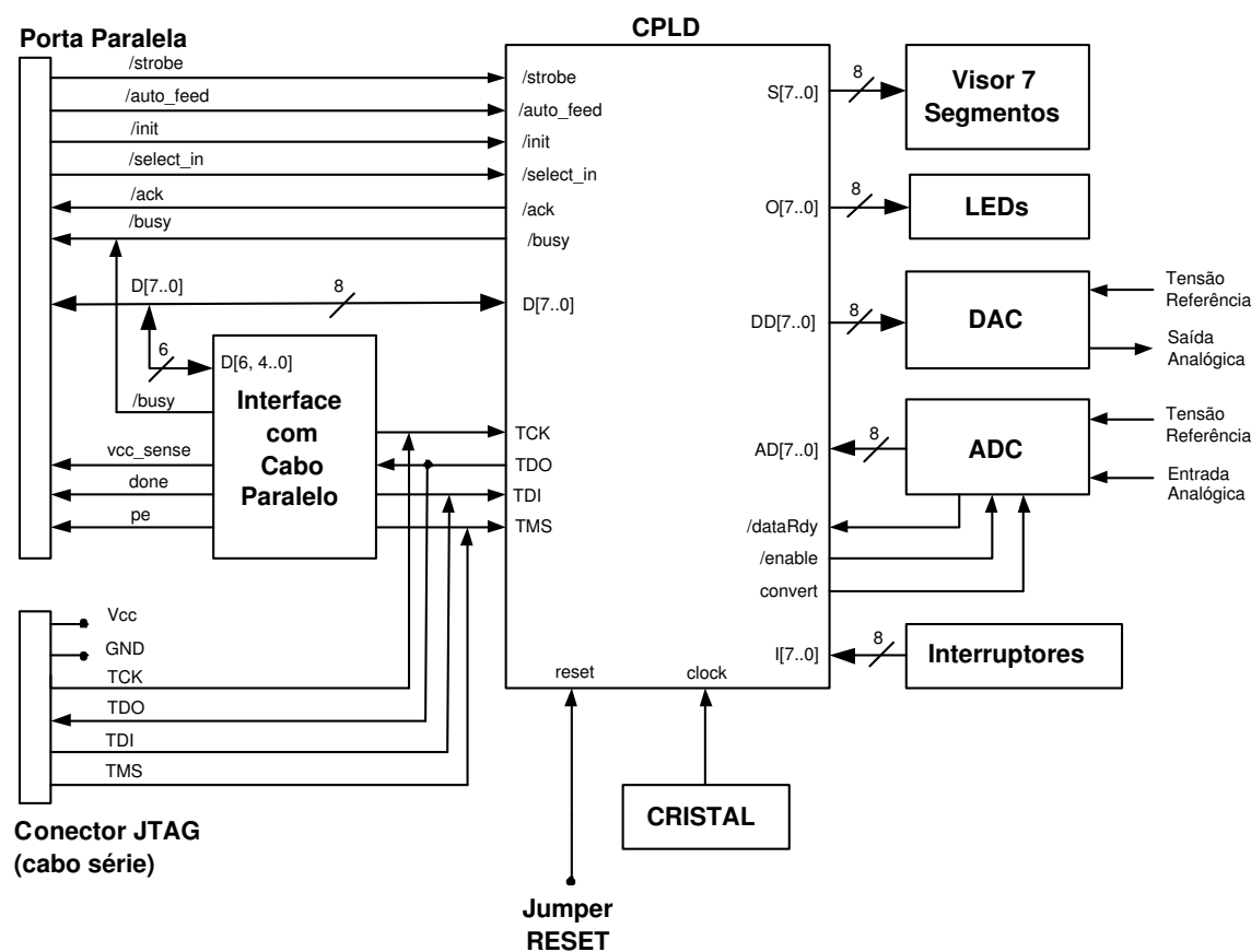
Figura 22: Diagrama de blocos simplificado do PG04 versão 2.
