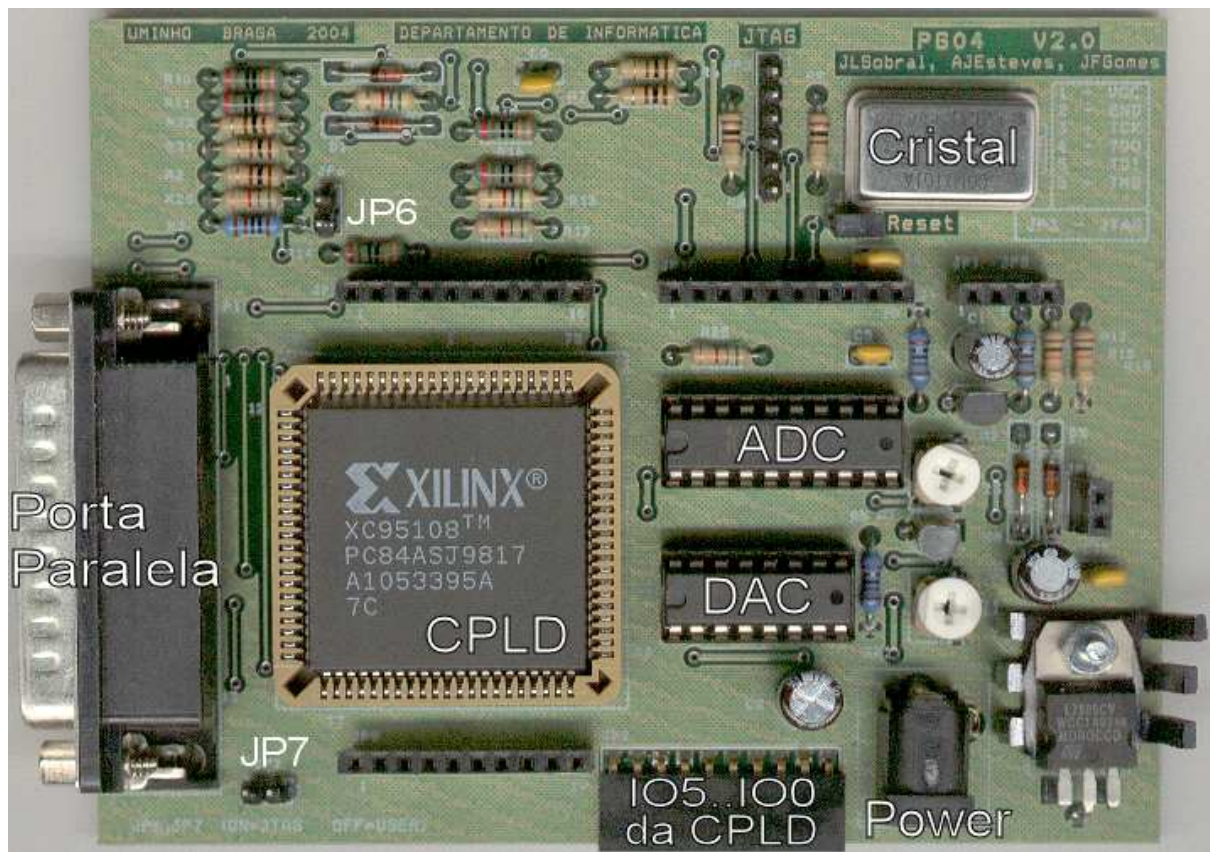
Figura 23: Placa principal do PG04 versão 2.
